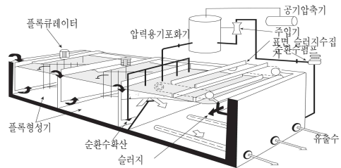
그림 4.5-1 일반적인 용존공기부상 공정도
