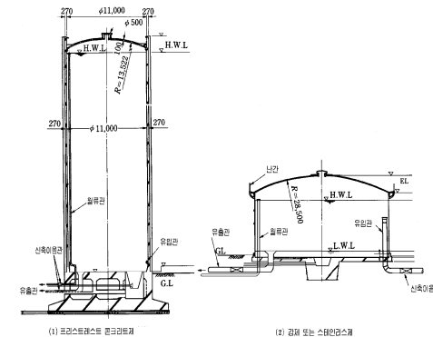
그림 4.2-1 배수탑의 예
