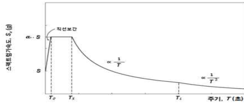
그림 4.1-1 암반지반 수평설계지반운동의 가속도 표준설계응답스펙트럼(5 % 감쇠비)
