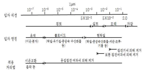
그림 4.3-1 수중에 존재하는 물질과 적용처리법
