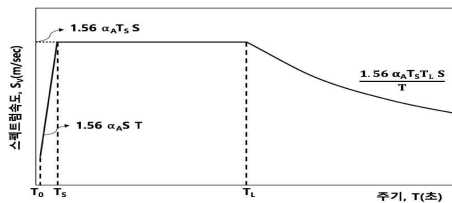
그림 4.1-2 암반지반(기반암) 평설계지반운동의 속도 표준설계응답스펙트럼(5 % 감쇠비)
