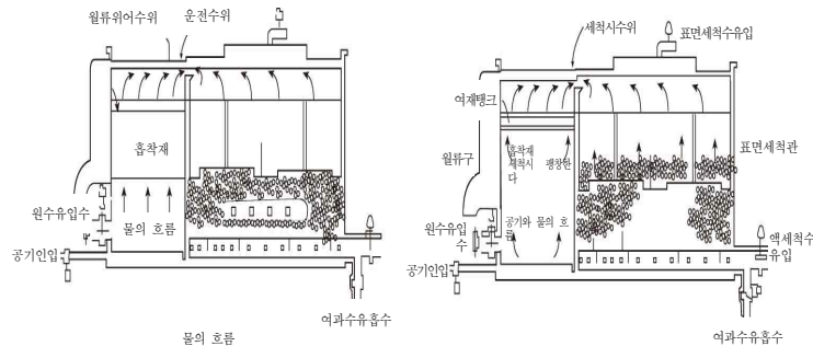
[그림 4.6-2] 실용화된 2단여과방식(인용 : Neptune Microfloc, Inc.)
