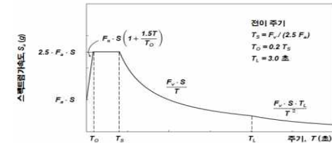
그림 4.1-3 토사지반 수평설계지반운동의 가속도 표준설계응답스펙트럼(5 % 감쇠비)
