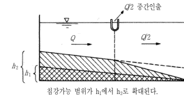
그림 4.4-3 중간 인출식 침전지의 효과
