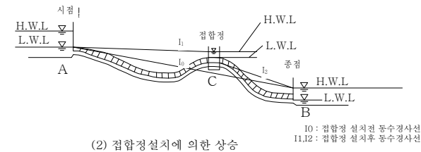
그림 4.1-2 동수경사선의 상승 사례
