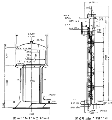
그림 4.2-2 배수탑의 예
