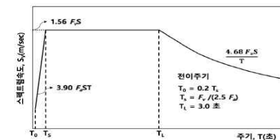
그림 4.1-4 토사지반 수평설계지반운동의 속도 표준설계응답스펙트럼(5 % 감쇠비)
