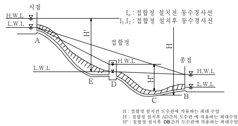
그림 4.1-3 도수관에서 정수압의 경감 사례
