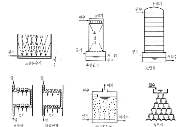
그림 4.12-1 폭기설비의 예
