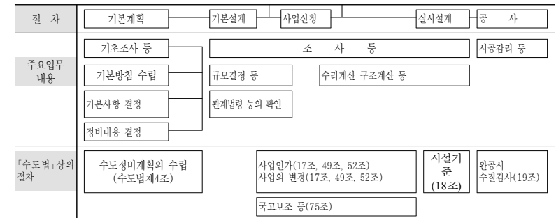
그림 1.6-1 상수도시설의 기본계획 및 정비절차
