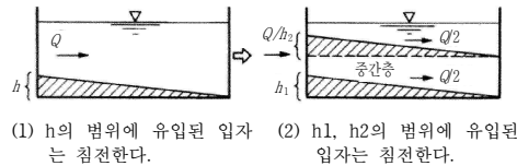
그림 4.4-2 2층식 침전지의 효과
