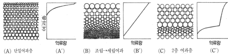
그림 4.6-1 여과층의 입도분포와 탁질억류량 분포
