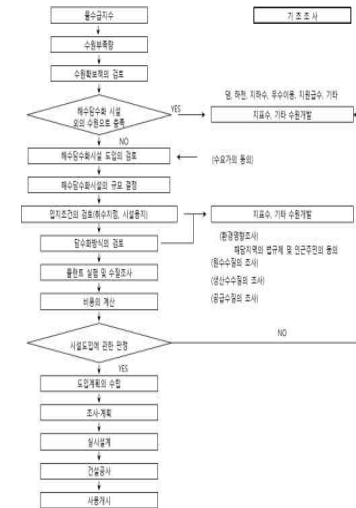
그림 4.21-1 해수담수화시설 도입과정의 흐름도
