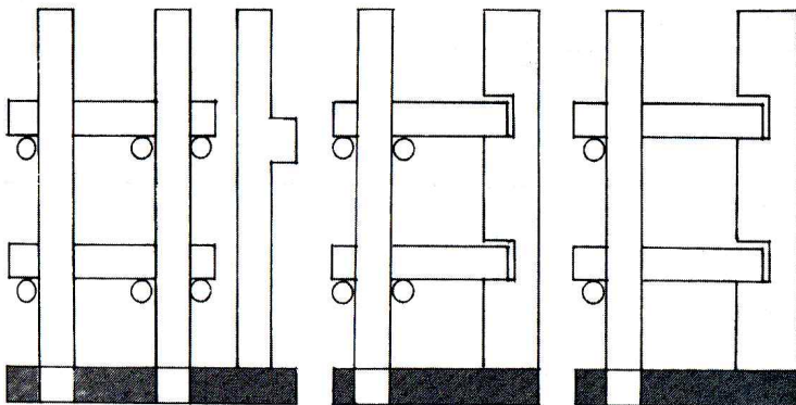
쌍줄비계
