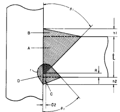
(8) 베벨형 T이음용접
