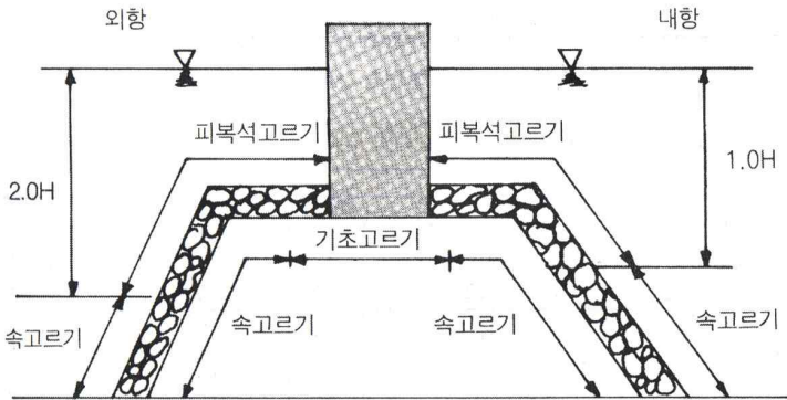
※ H는 설계파고
