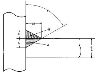
(10) 베벨형 필릿 T이음용접
