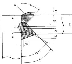
(7) K형 모서리이음용접
