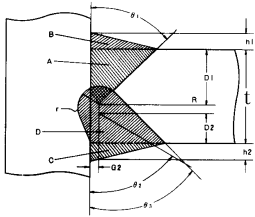
(9) K형 T이음용접
