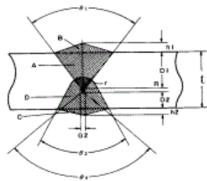
(5) X형 판이음용접
