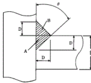
(13) 베벨형 부분용입과 모서리이음용접의 병용
