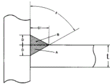
(10) 베벨형 필릿 T이음용접
