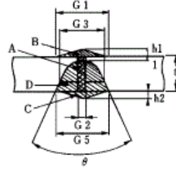
(2) I형 판이음용접
