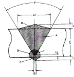
(4) V형 판이음용접
