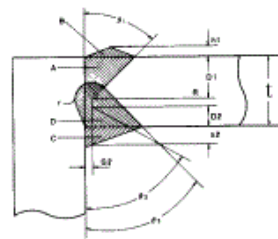
(7) K형 모서리이음용접
