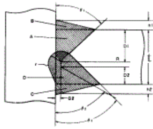
(9) K형 T이음용접
