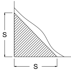
(1) 필릿용접
