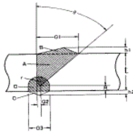
(3) 베벨형 판이음용접
