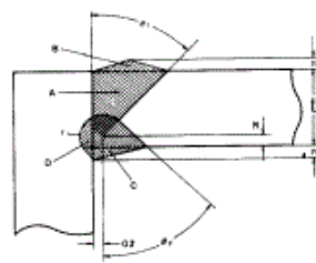
(4) V형 판이음용접
