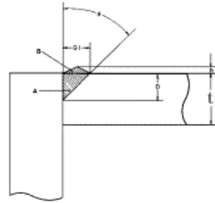
(12) 베벨형 부분용입 모서리이음용접
