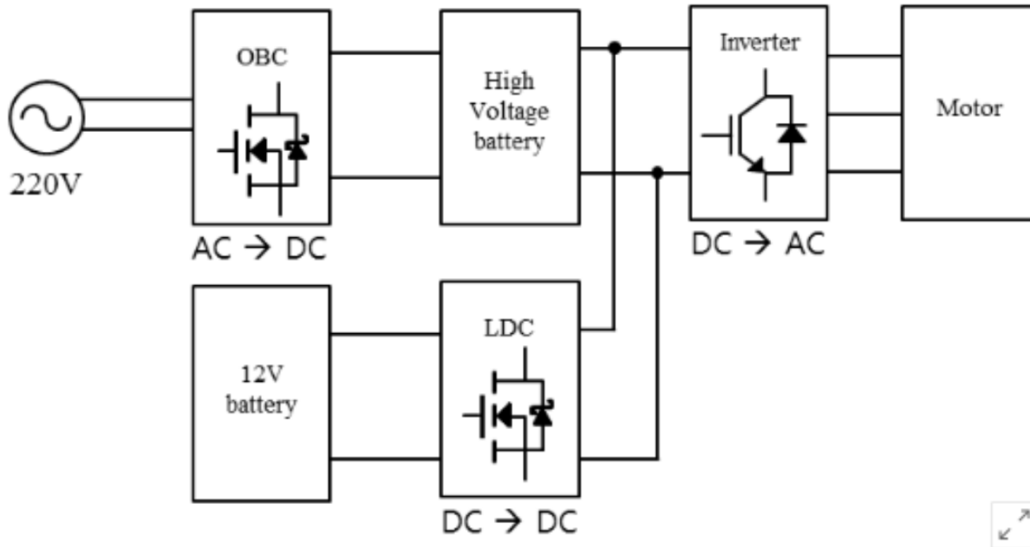
전력변환장치의 구성도
