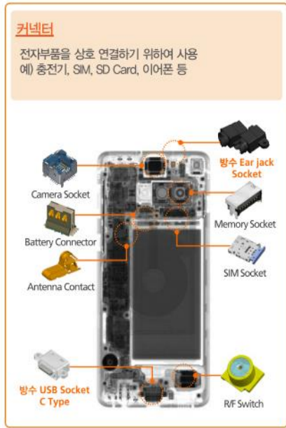
도표 25. 방수, 고속(C Type), 5G 등 최신 모바일 트렌 변화에 맞춘 고기능성 커넥터 생산
